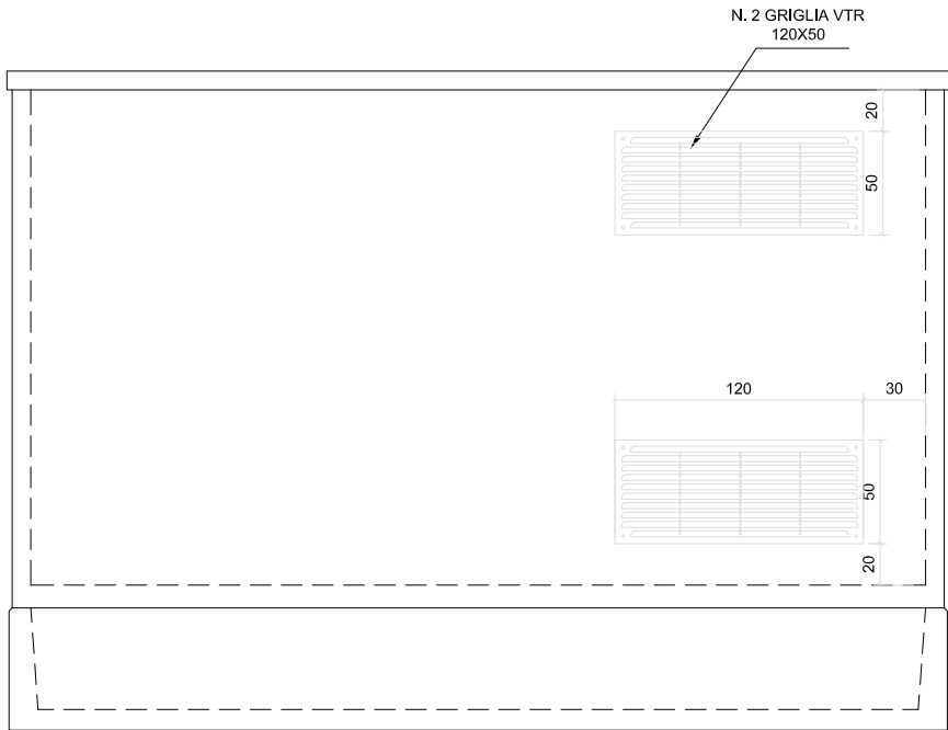
VISTA LATO POSTERIORE
