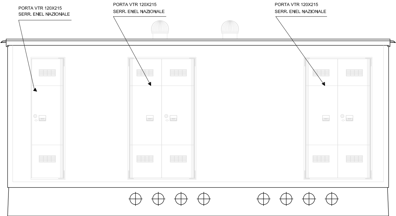
VISTA LATO FRONTALE
