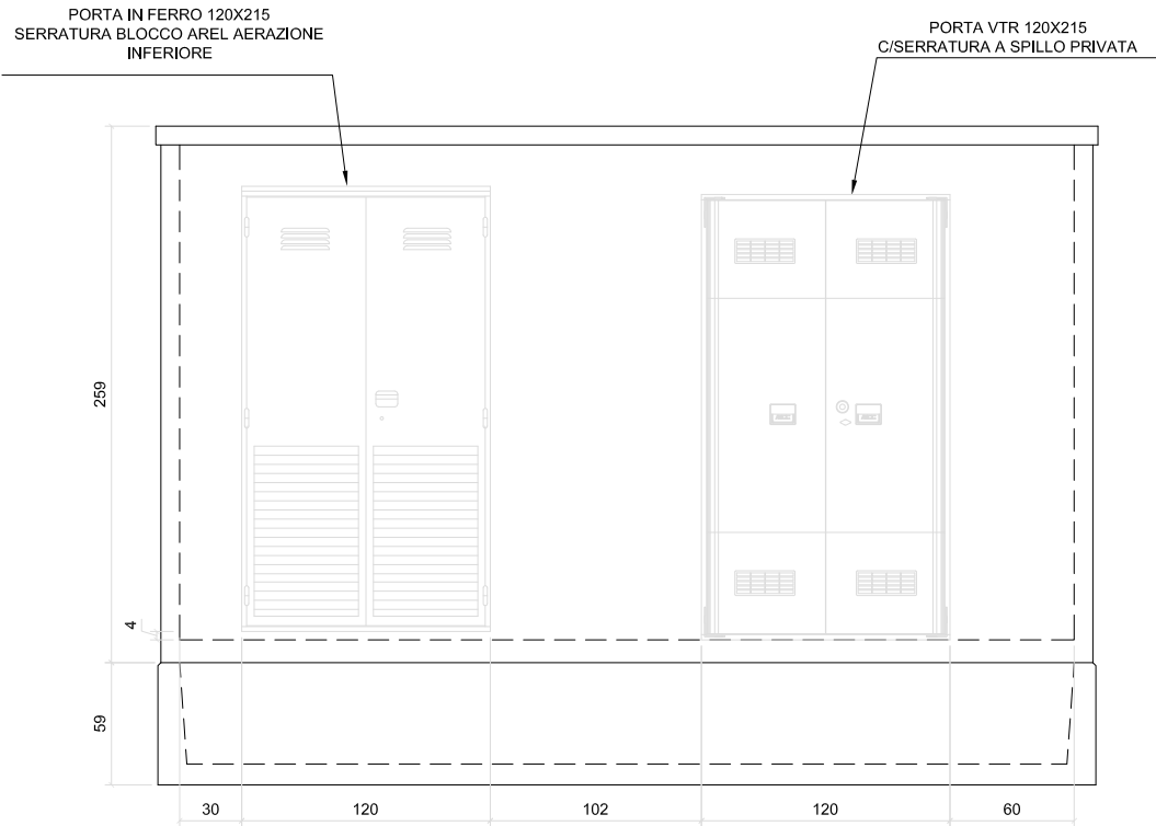
VISTA LATO FRONTALE
