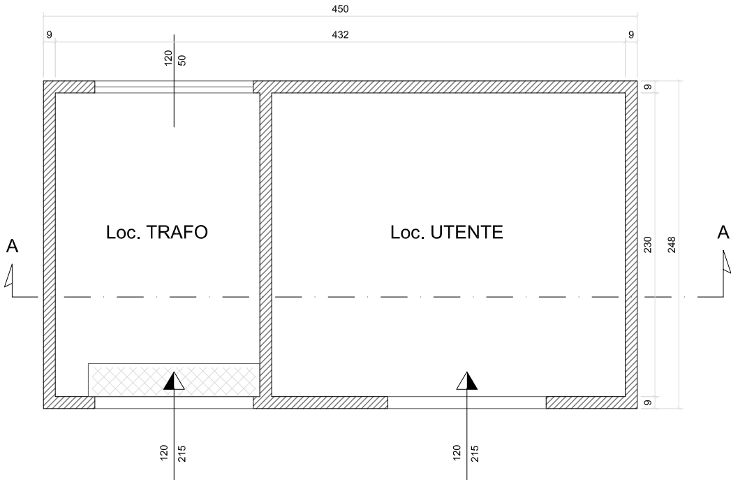
PIANTA
