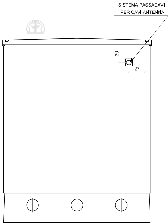
VISTA LATO DESTRO
