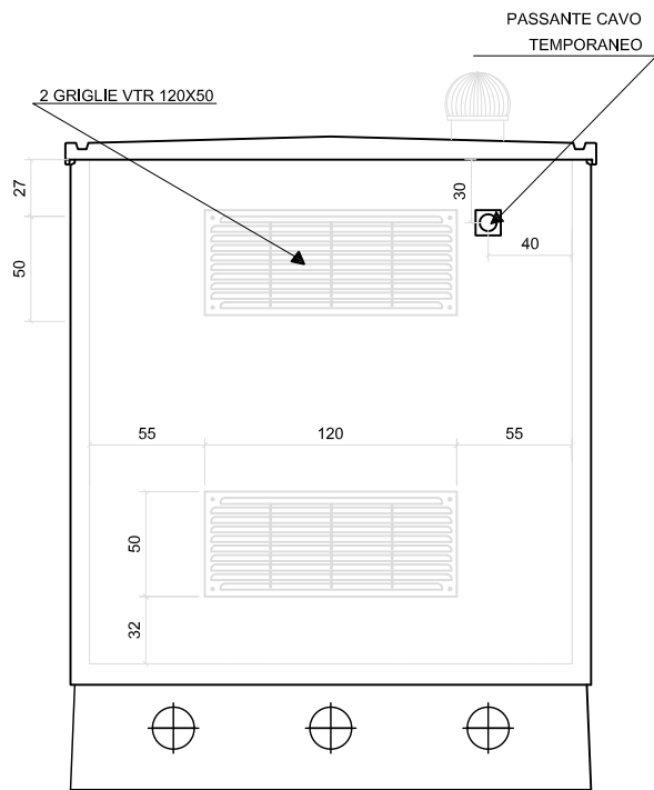
VISTA LATO SINISTRO
