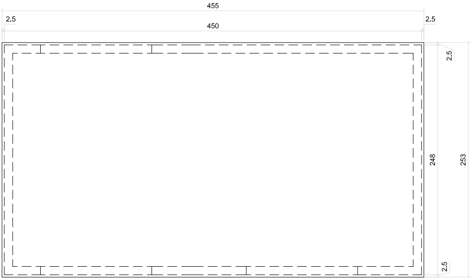
PIANO COPERTURA
